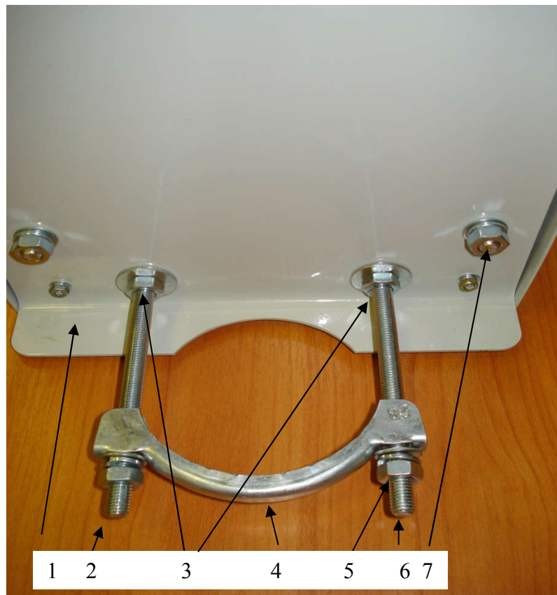
Рис. 2 - Узел крепления БПЭС. 1 – шасси БП; 2, 6 – болты крепления; 3 – гайки крепления болтов; 4 – скоба, 5 – гайки крепления скобы, 7- крепеж шасси.
